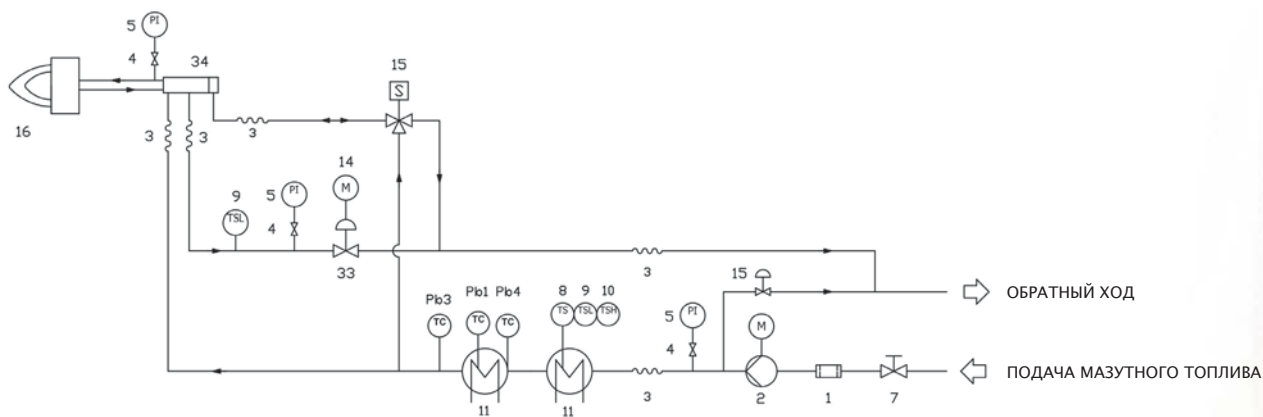
Сх.01 – Схема для мазутного топлива: пример с горелками серии PN, KP одnogоловочными
