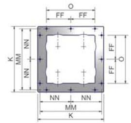
Фланец горелки
