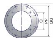
контрфланец
