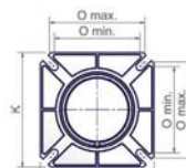
Фланец горелки
